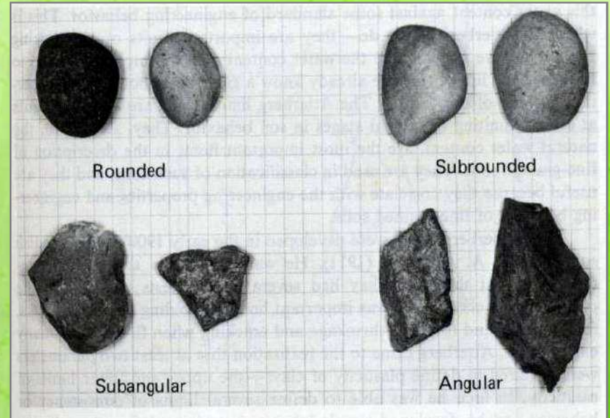
Bentuk Tipikal Butiran Kasar
