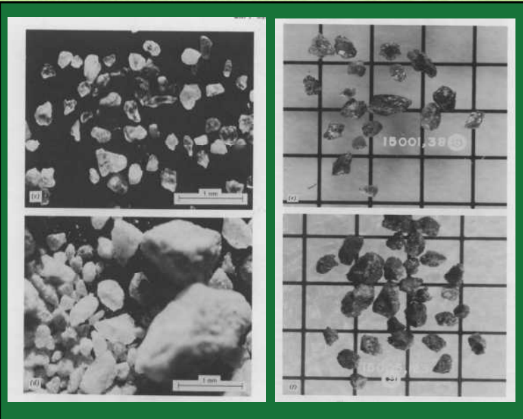
Bentuk Tipikal Butiran Kasar
